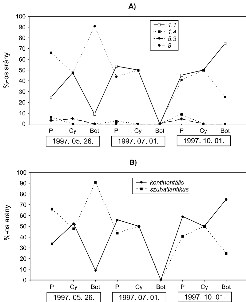
3. ábra. Állatföldrajzi megoszlás A – faunakörök, B – kontinentális, szubatlanti faunakör csoportok P=Achilleo-Festucetum pseudovinae; Cy=A.-F. cydonetosum; Bot=A.-F. bothriochloetosum
