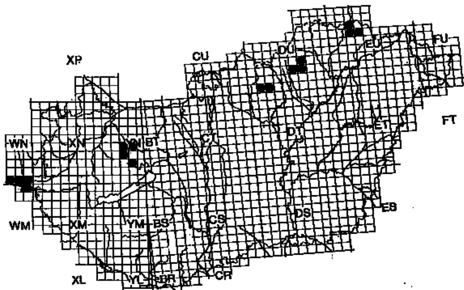
1. ábra: Triturus alpestris lelőhelyek elhelyezkedése Magyarország UTM rendszerű térképén
