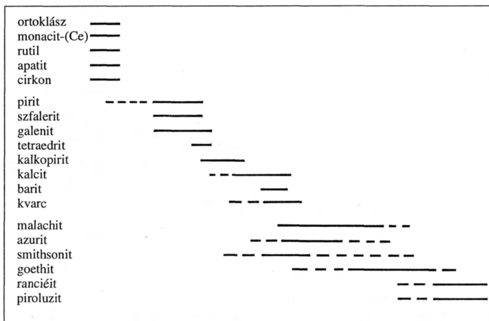
8. ábra. A rakacsazendi ércindikáció ásványainak kiválási sorrendje. Succession of minerals of of Rakacsazend ore indication
